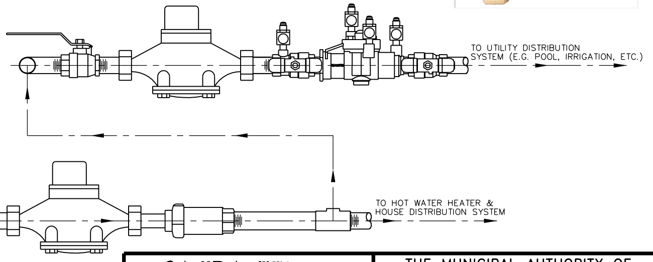
ELEVATION
